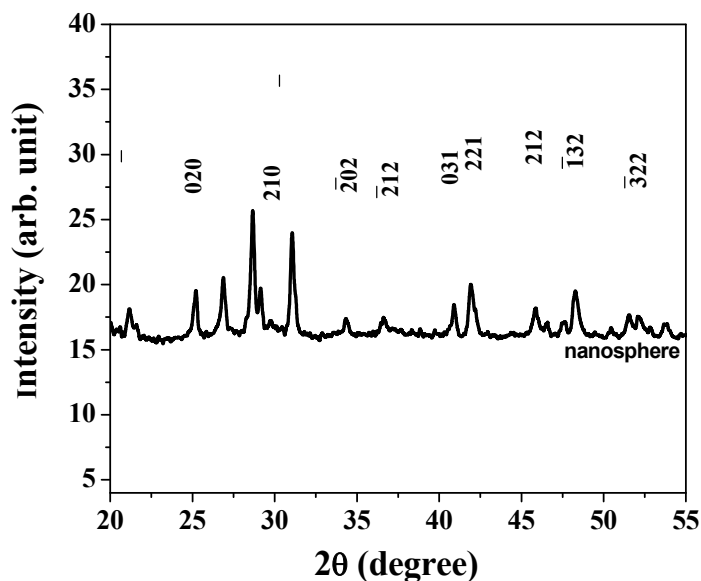
Fig.1: XRD of BAM:Eu
