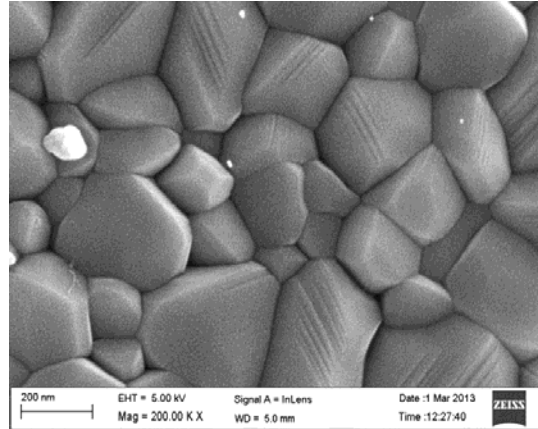
Fig.1: HRSEM of BAM:Eu
